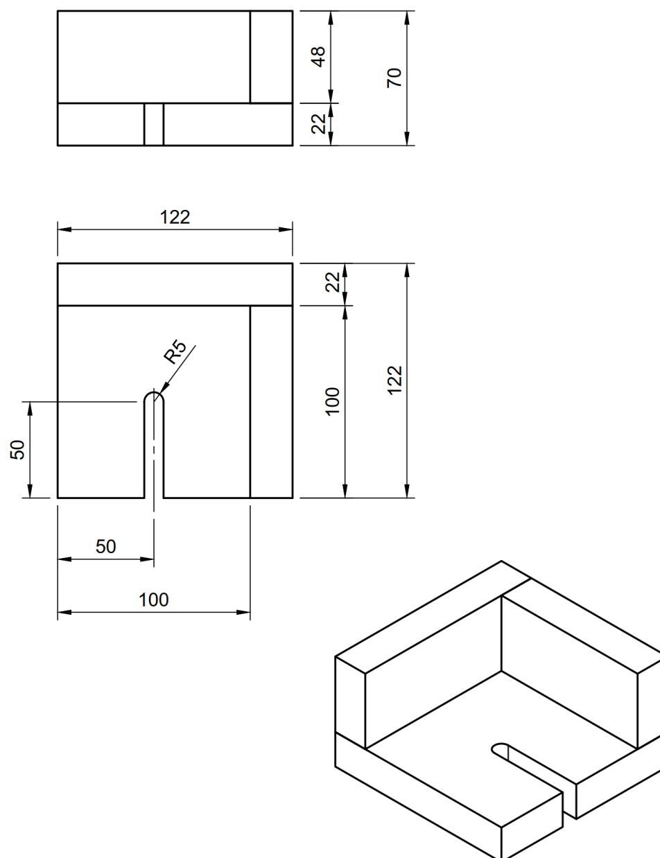
FIGURE 33 – Support de balise fixe droit
