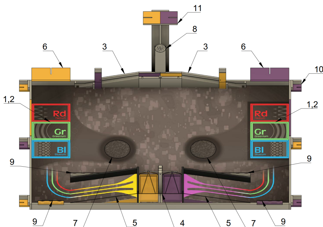
FIGURE 4 – Vue détaillée de l'aire de jeu
