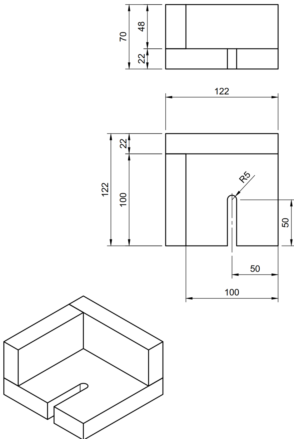
FIGURE 32 – Support de balise fixe gauche
